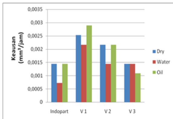
Gambar 5. Perbandingan Harga Keausan Wipro Untuk Berbagai Media Pembasahan
