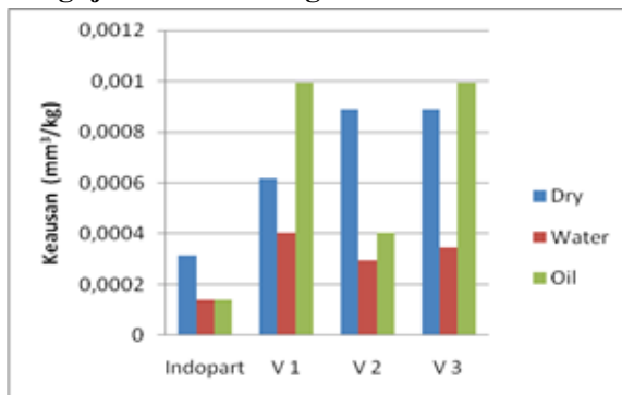
Gambar 4. Grafik Hasil Pengujian Keausan Ogohosi Untuk berbagai MediaPembasahan Pengereman
