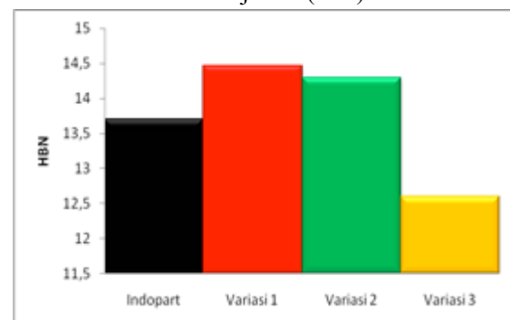
Gambar.3. Harga Kekerasan Variasi Kampas Rem.
